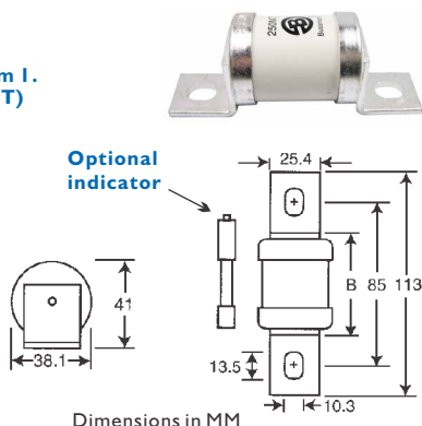
Diagram 2. (FMM / MMT)
